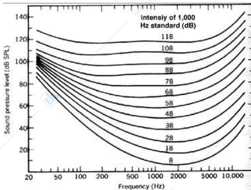
Figura 2.27: Curve di eguale intensità percepita (Fletcher and Munson, 1933)
