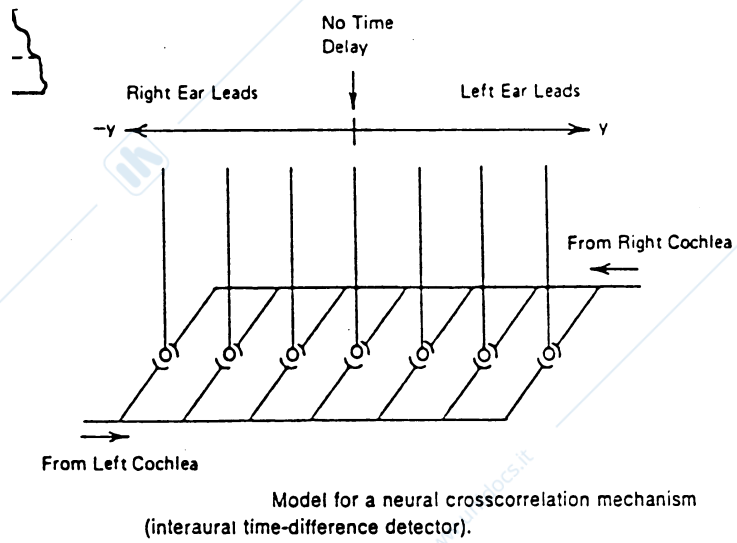
Figura 2.24: Modello di individuatore di differenze temporali interaurali
