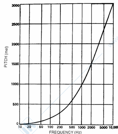
Figura 2.9: Scala mel
