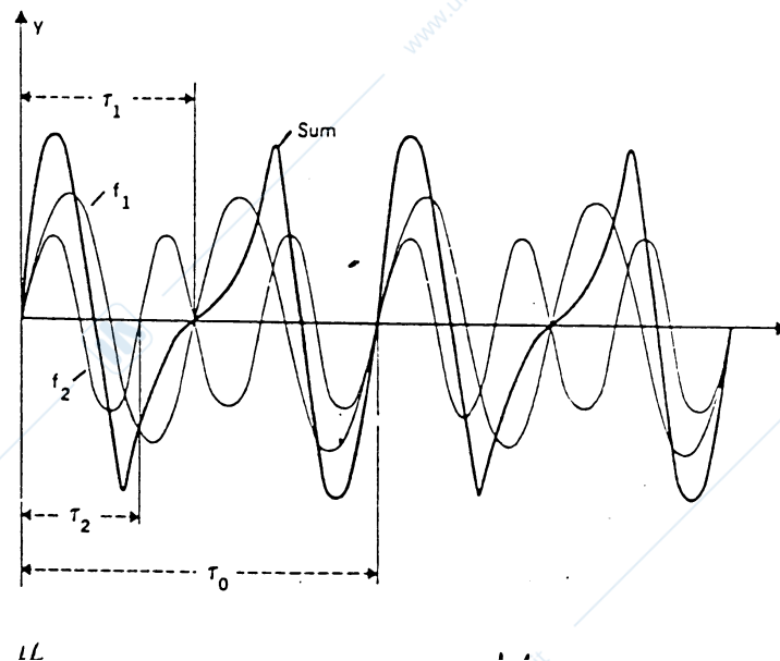
Figura 2.20: Ricostruzione della fondamentale ( \tau_1 = \frac{1}{f_1} , \tau_2 = \frac{1}{f_2} , \tau_0 = \frac{1}{f_0} )
