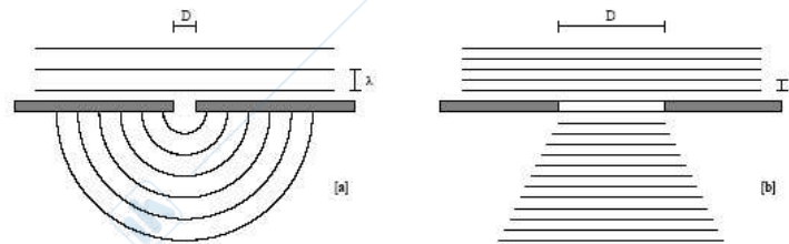
Figura 2.3: Effetto della diffrazione nei casi \lambda > D in [a] e \lambda < D in [b]
