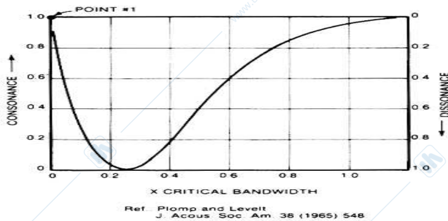
Figura 2.16: Consonanza (e dissonanza) tra due toni al variare della loro separazione in frazione di larghezza di banda critica.
