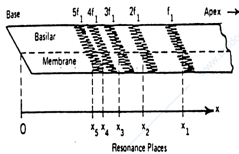
Figura 2.25: Pattern spaziale sulla membrana basilare dovuto a un suono armonici
