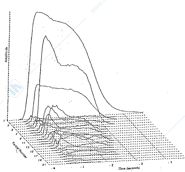
Figura 2.32: Rappresentazione tempo-frequenza-ampiezza di un suono
