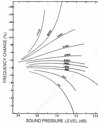
Figura 2.11: Diagramma di Stevens e Wolkman (1937). Variazione del pitch di una sinusoide in funzione dell'intensità. Una sinusoide di 150 Hz passando da 45 a 90 dB scende in pitch del 12%, circa di due semitoni. Una curva discendente implica che la frequenza del suono deve essere aumentata per avere la stessa sensazione di pitch.
