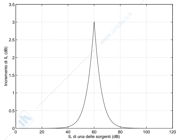
Figura 2.4: Incremento del livello di intensità, rispetto la sorgente di intensità maggiore, nel caso di due sorgenti, la prima fissa a 60 dB e la seconda variabile da 0 dB a 120 dB
