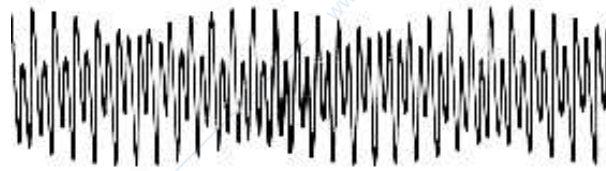
Figura 2.18: Esempio di battimenti del II ordine tra 100 e 201 Hz (frequenza di battimento 1 Hz).
