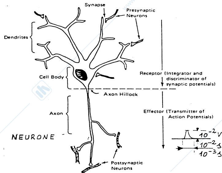
Figura 2.21: Neurone
