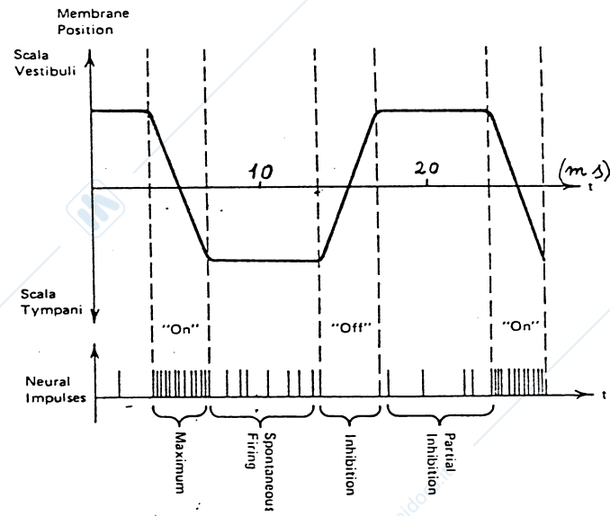
Figura 2.22: Treno di impulsi generato da un'onda periodica
