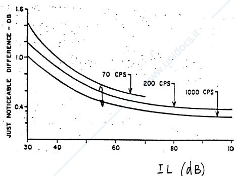
Figura 2.26: Valori di JND di intensità per valori diversi di IL e frequenza del suono puro
