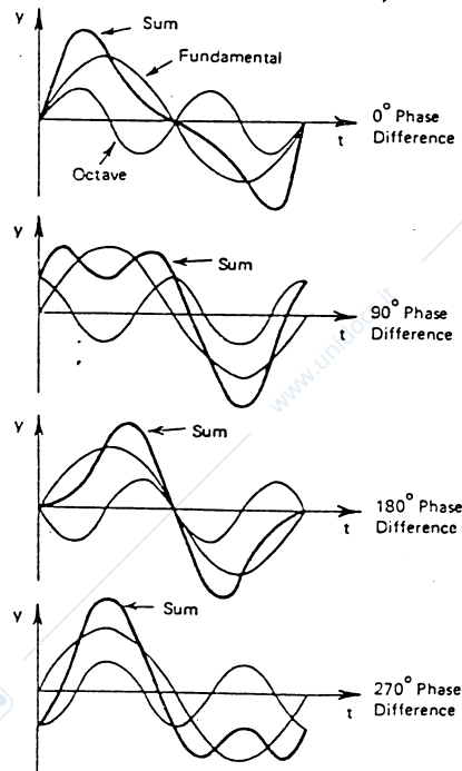
Figura 2.18: Esempio di battimenti del II ordine tra 100 e 201 Hz (frequenza di battimento 1 Hz).
