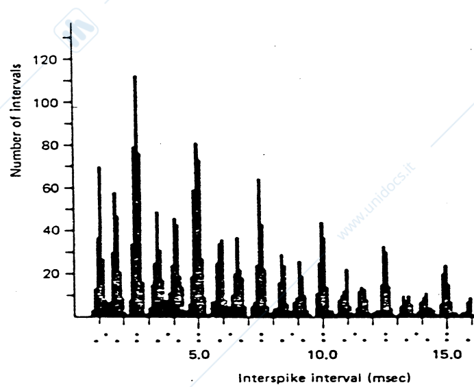
Figura 2.23: Istogramma del numero di occorrenze di dato tempo di intercorrenza fra spike successivi nel nervo uditivo a fronte di un'eccitazione composta da due suoni puri
