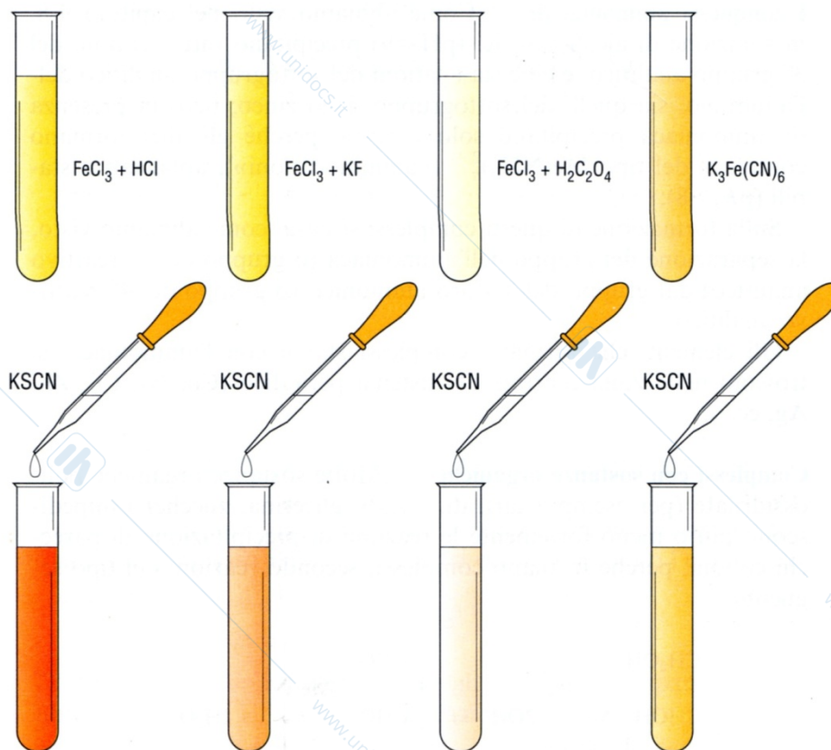
FIGURA13-8 L'effetto mascherante dei complessi. Soluzioni di ioni Fe 3+ contenenti vari complessanti vengono trattate con KSCN; il composto Fe(SCN) 3 di colore rosso vivo si forma più facilmente nella soluzione cloridrica.
