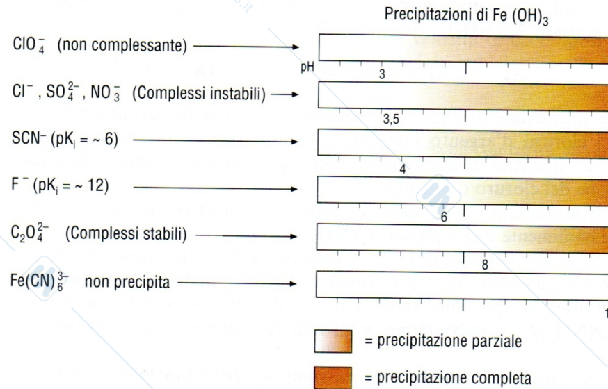
FIGURA 15-1 Il pH di precipitazione di Fe(OH) 3 in presenza di vari complessanti.
