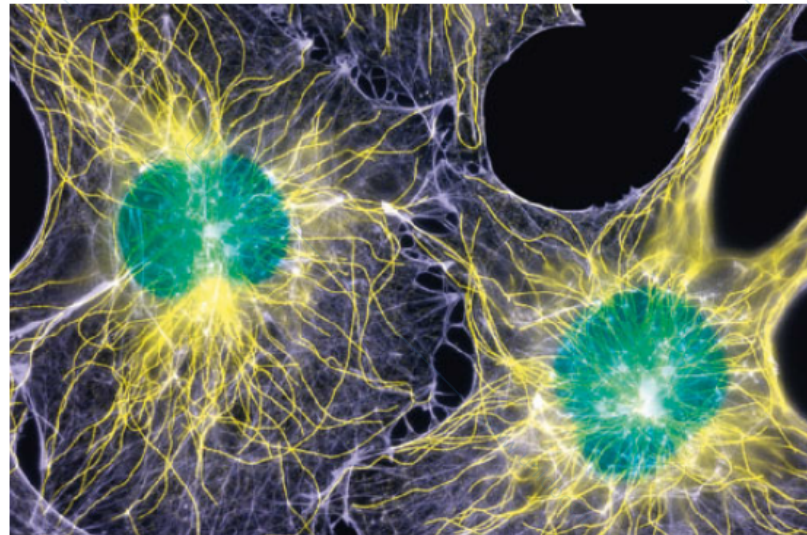
Cellule in cui sono evidenti i microtubuli (in giallo) che formano il citoscheletro, visibili grazie alla tecnica della microscopia a fluorescenza.
