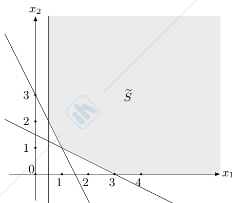
Figura 5.10: La regione ammissibile \tilde{S}
