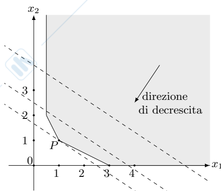
Figura 5.11: Curve di livello della funzione 400x_1 + 600x_2 e punto di ottimo
