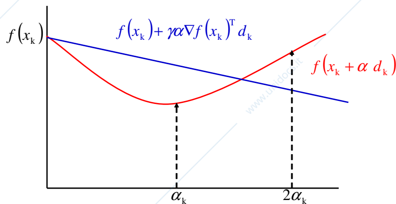
Figura 2.2: Esempio di un passo \alpha_k .
