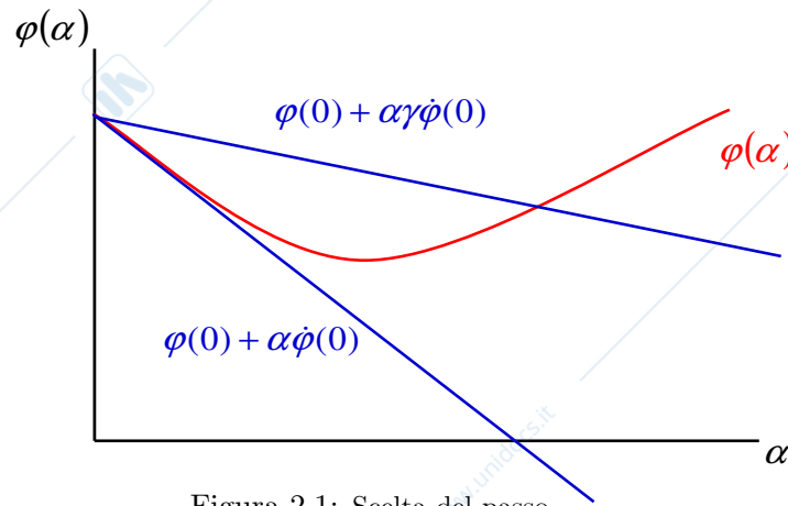
Figura 2.1: Scelta del passo.
