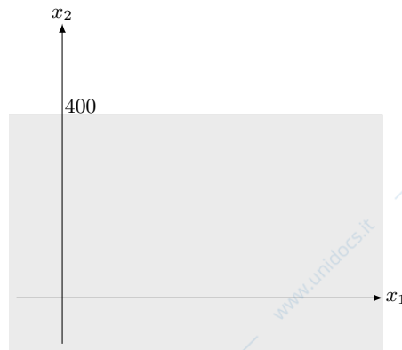
Figura 5.3: Semipiano individuato dal vincolo x_2 \leq 400
