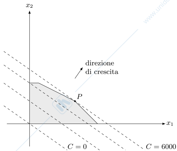
Figura 5.5: Curve di livello della funzione f(x_1, x_2) = 7x_1 + 10x_2 e punto di ottimo
