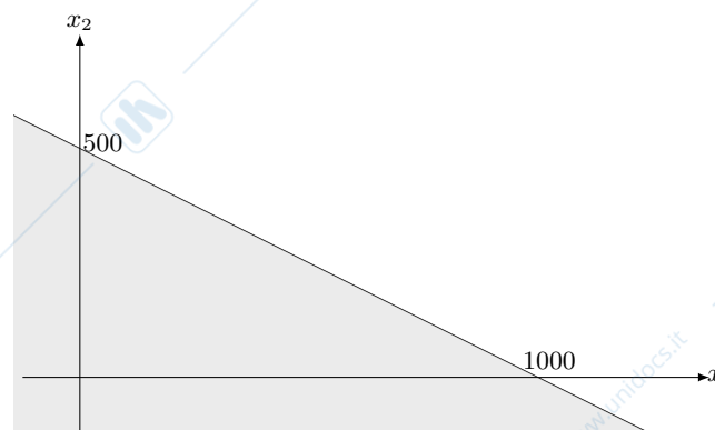
Figura 5.2: Semipiano individuato dal vincolo x_1 + 2x_2 \leq 1000
