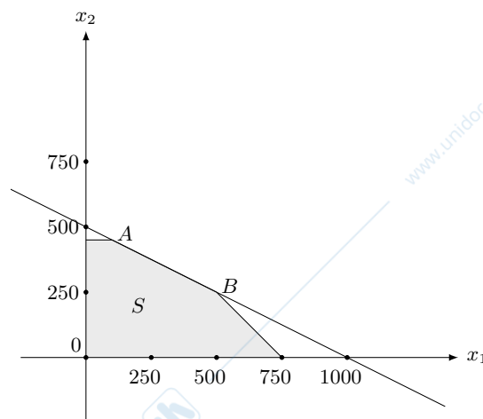
Figura 5.6: Esempio di soluzione non unica
