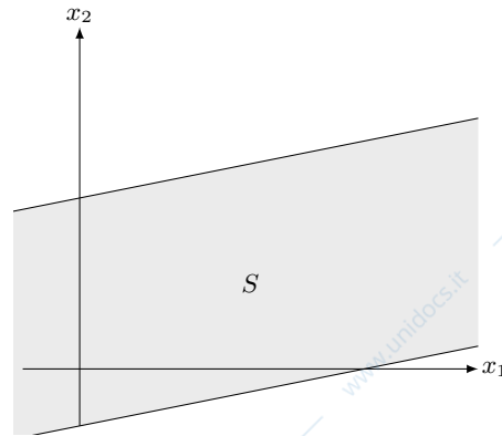
Figura 5.12: Regione ammissibile costituita da una striscia di piano
