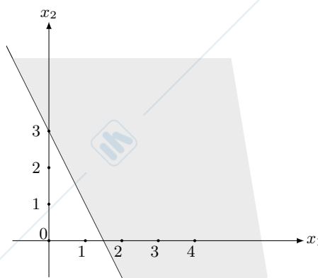
Figura 5.8: Semipiano individuato dal vincolo 20x_1 + 10x_2 \geq 30
