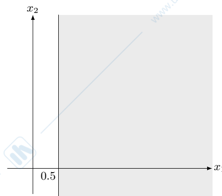
Figura 5.7: Semipiano individuato dal vincolo 140x_1 \geq 70
