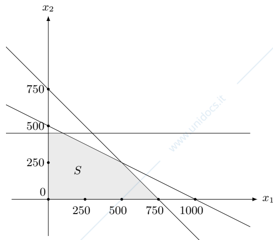
Figura 5.4: La regione ammissibile S
