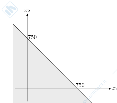
Figura 5.1: Semipiano individuato dal vincolo x_1 + x_2 \leq 750
