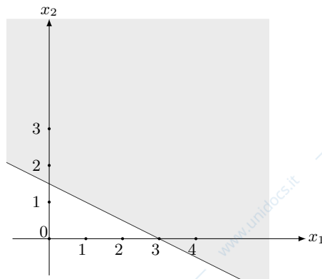
Figura 5.9: Semipiano individuato dal vincolo 25x_1 + 50x_2 \geq 75
