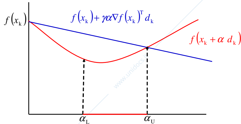
Figura 2.3: Intervallo di accettabilità per \alpha_k .
